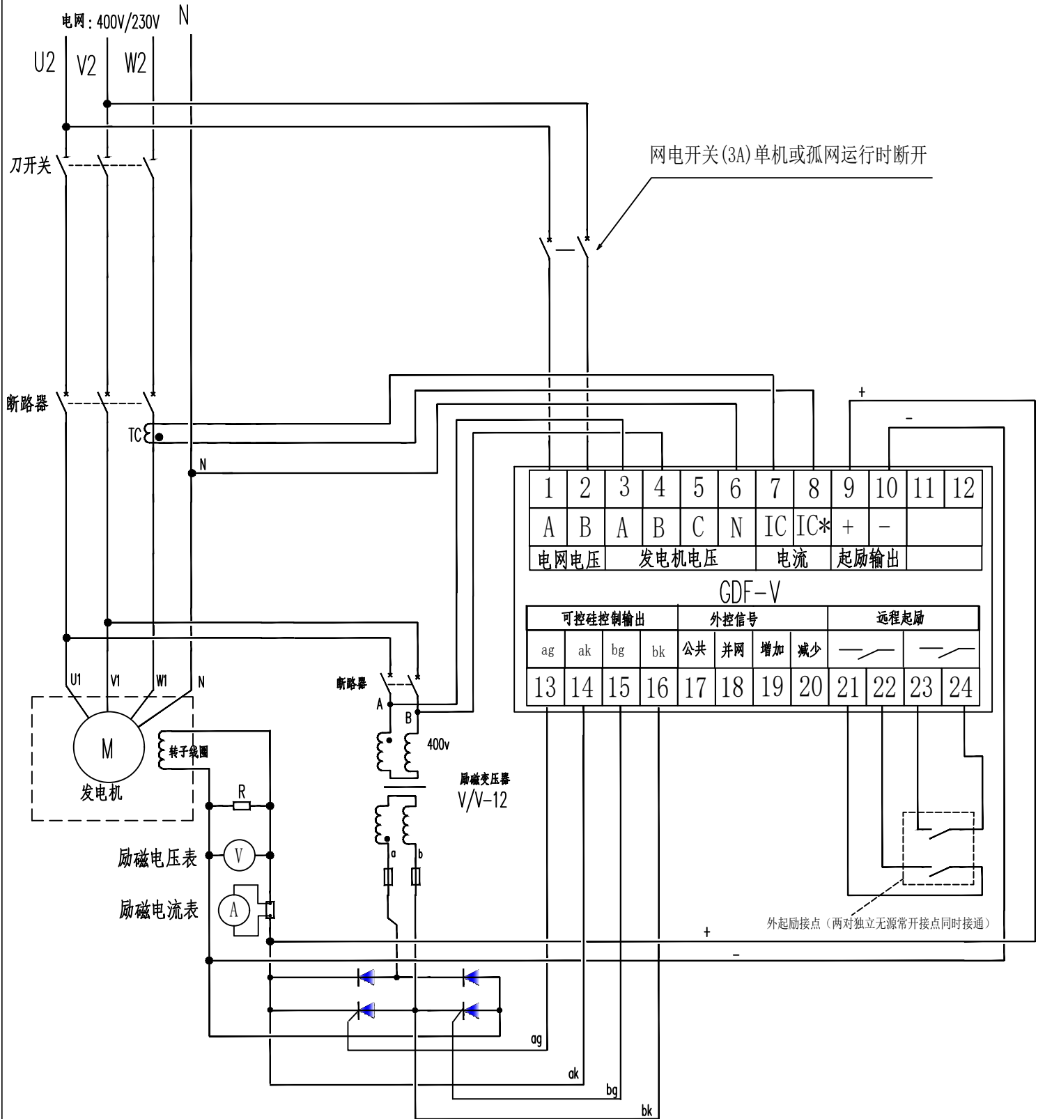
附图2: V型控制器外接线图 (可控硅两个首尾串接)
