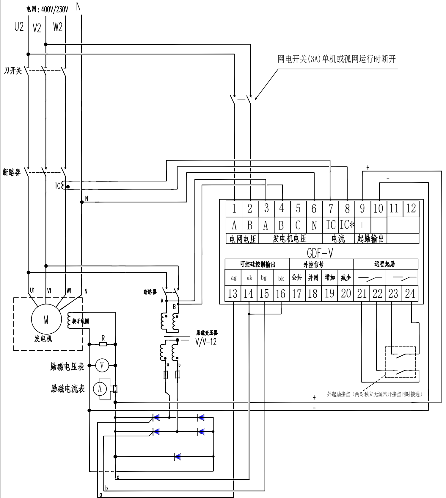
附图1: V型控制器外接线图 (可控硅二相共阴极)
