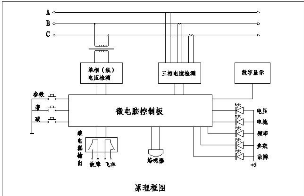
图 6 原理框图
